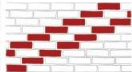
Ложковая диагональная со сдвигом в четверть кирпича
