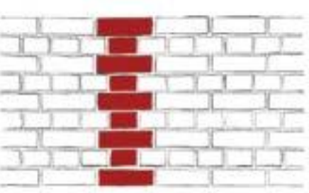
Крестовая. Тип II
