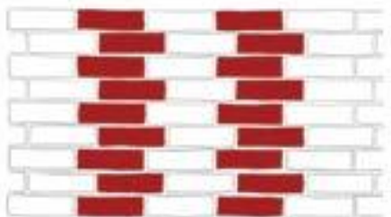
Ложковая в четверть кирпича
